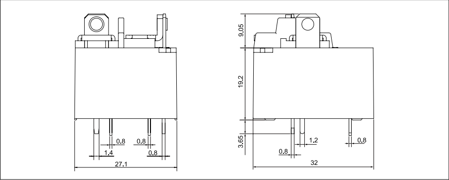
外形尺寸 OUTLINE DIMENSIONS
