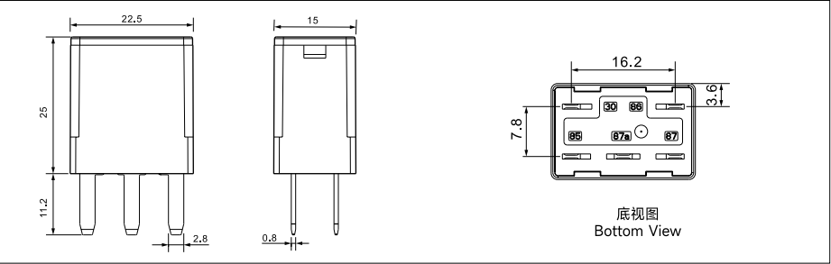
外形尺寸 OUTLINE DIMENSIONS
