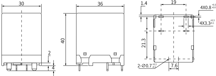
外形尺寸 Outline Dimensions
